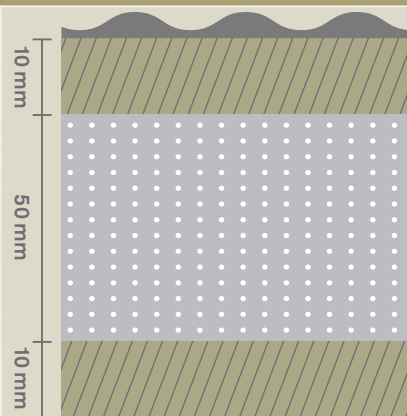
Querschnitt der Kuschelmatte
